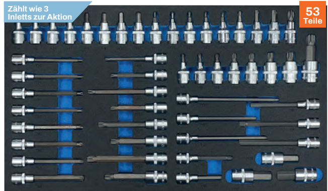
Steckschlüssel-Einsätze 1/2" TX Gr. 20 – 55, Vielzahn Gr. 5 – 18 mm, Innen-6-kant Gr. 5 – 19 mm
