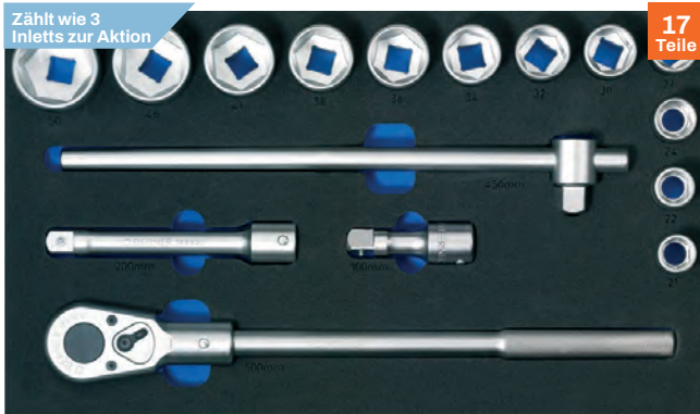
Steckschlüssel-Satz 3/4" SW 21 – 50 mm*
